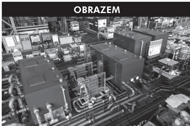
Na montáži haly pět právě v těchto dnech probíhá montáž hydraulické části kovového lisu CKW 3300/4000 pro japonského zákazníka Nakamura Iron Works. Montáž mechanické části bude následovat v letních měsících. Prestižní zakázku v hodnotě téměř 200 milionů korun získal ŽDAS loni v březnu.
