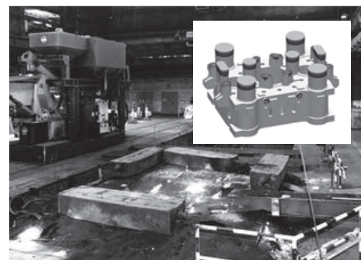
V noci na středu 13. června byl v provozu metalurgie vyroben odlitek horní traverzy o surové hmotnosti 77 350 kg pro projekt Bonatrans. Výrobě předcházela simulace pomocí softwaru Magma.
