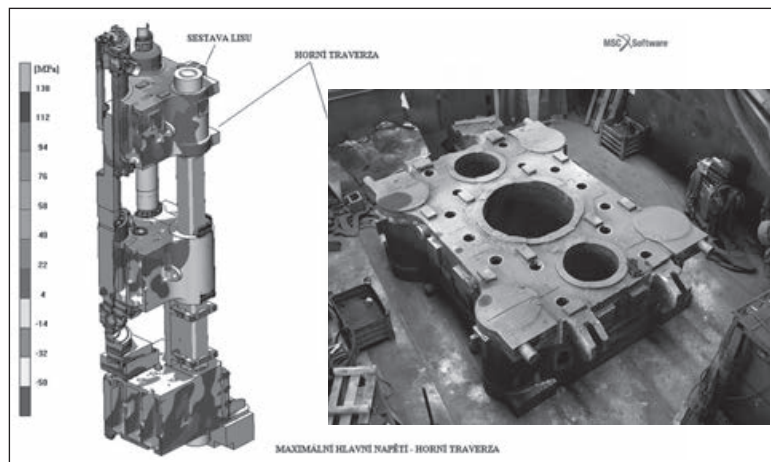
Jeden z výsledků simulace symetrického zatížení budoucího lisu (řez, jedna čtvrtina) a fotografie současného stavu odlitku horní traverzy
