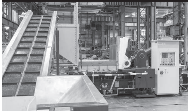
Na montáži haly 4 probíhala v červnu a červenci montáž linky s lísou CPB 100 pro firmu MORAVIA CANS a.s. Bojkovice. V současné době je lis již demontován a bude následovat expedice. Linka s lísou CPB 100 je určena k paketování zmetkových dílů a výrobního odpadu při výrobě aerosolové hliníkové nádoby pro kosmetický, chemický a farmaceutický průmysl.
