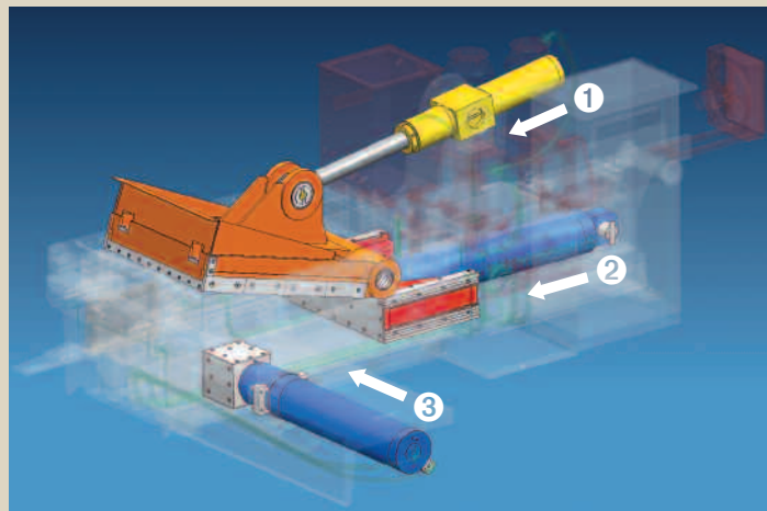
Schéma hydraulických částí lisu CPB
